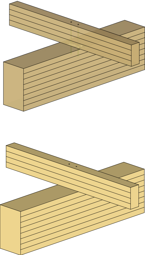
A.07 Fixação do barrote sobreposto na viga
