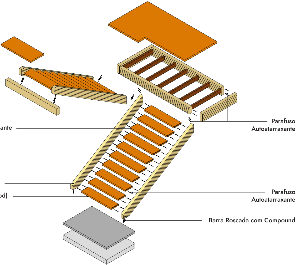
D.01 Escada padrão 2 lances
